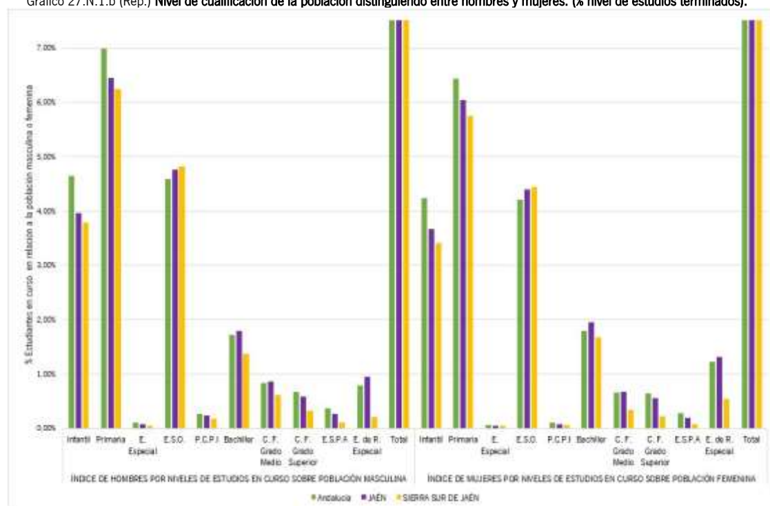
Gráfico 27.N.1.b (Rep.) Nivel de cualificación de la población distinguiendo entre hombres y mujeres. (% nivel de estudios terminados).
