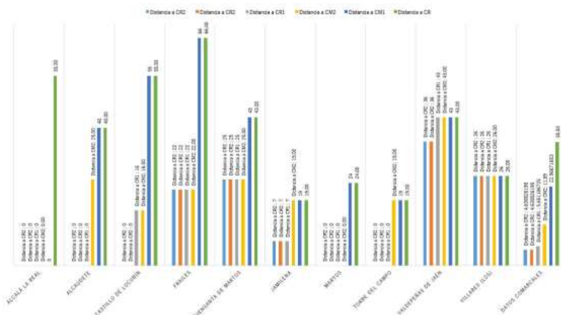
Gráfico 11. Duración del trayecto a ciudades con jerarquía en el Sistema de Ciudades del Plan de Ordenación Territorial de Andalucía (Unidad de medida: Minutos)
