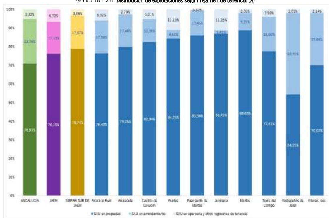
Grafico 18.L.2.d. Distribución de explotaciones según régimen de tenencia (%)
